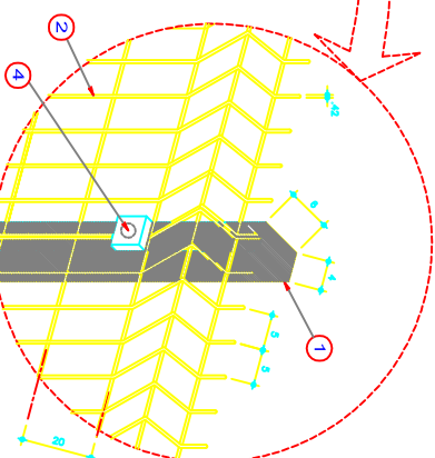
DET. 01 ESCALA: 1:5
